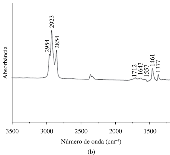
Figura 6. Espectros de infravermelho das amostras: a) não tratada; b) tratada durante 60 segundos.
