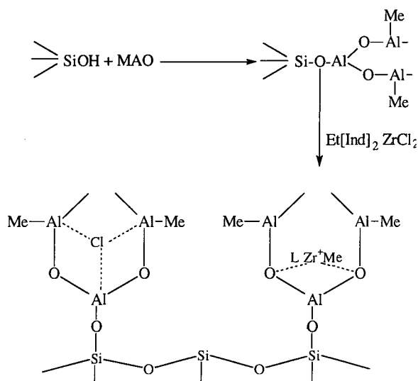
Figura 8. Formação de complexo do tipo coroa na superfície de suportes hidroxilados [25]
