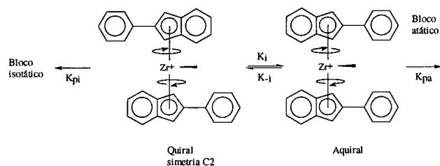
Figura 4. Complexo metalocênico com rotação entre os ligantes; catalisadores oscilantes [23, 33]
