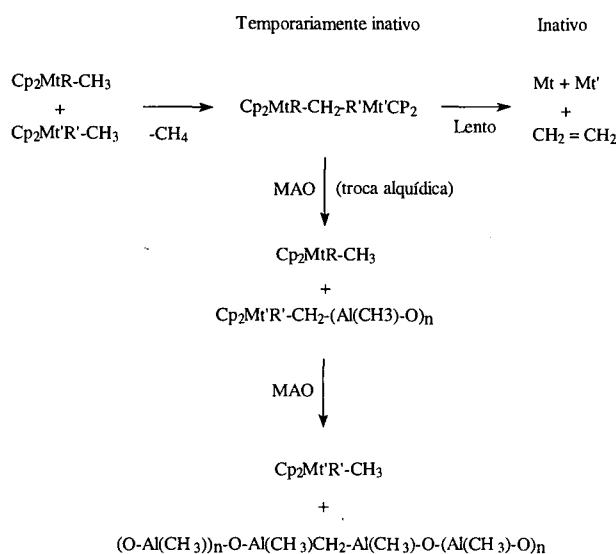
Esquema 2. Reações de desativação da espécie ativa do sistema metaloceno/MAO [23]
