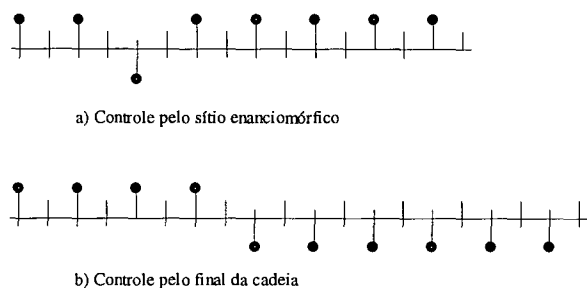
Figura 7. Microestrutura de polipropileno obtidas (a) por controle pelo sítio enantiomórfico e (b) por controle final da cadeia [21]
