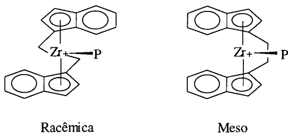
Figura 5. Formas isoméricas de catalisadores metalocênicos quirais [33]
