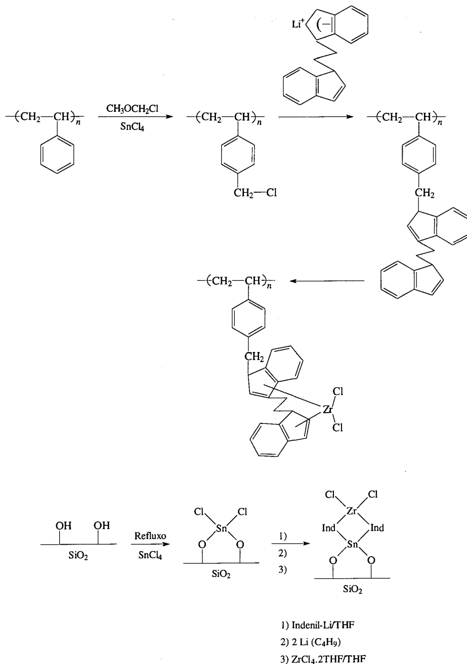
Figura 9. Exemplos de catalisadores metallocênicos suportados por ancoramento [52,55]
