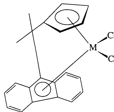
Figura 6. Estrutura de complexo metalocênico com simetria Cs [32]
