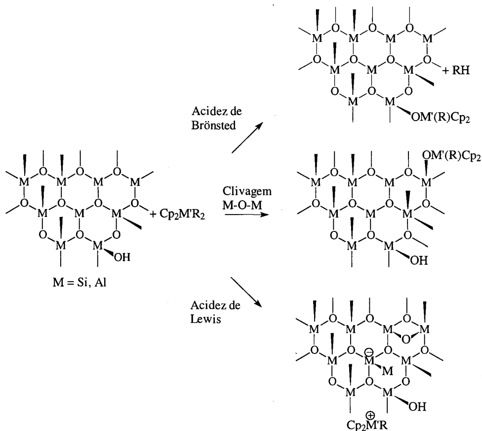
Figura 10. Reações possíveis do complexo metalocênico com a superfície de suportes do tipo óxidos inorgânicos [66]
