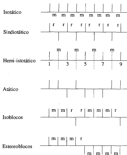
Figura 3. Algumas configurações possíveis para as cadeias de polipropileno [71]
