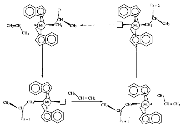
Figura 2. Mecanismos de Polimerização via sistema metaloceno/MAO [8]
