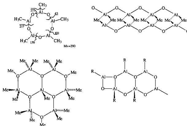
Figura 1. Algumas propostas [10] para a estrutura MAO
