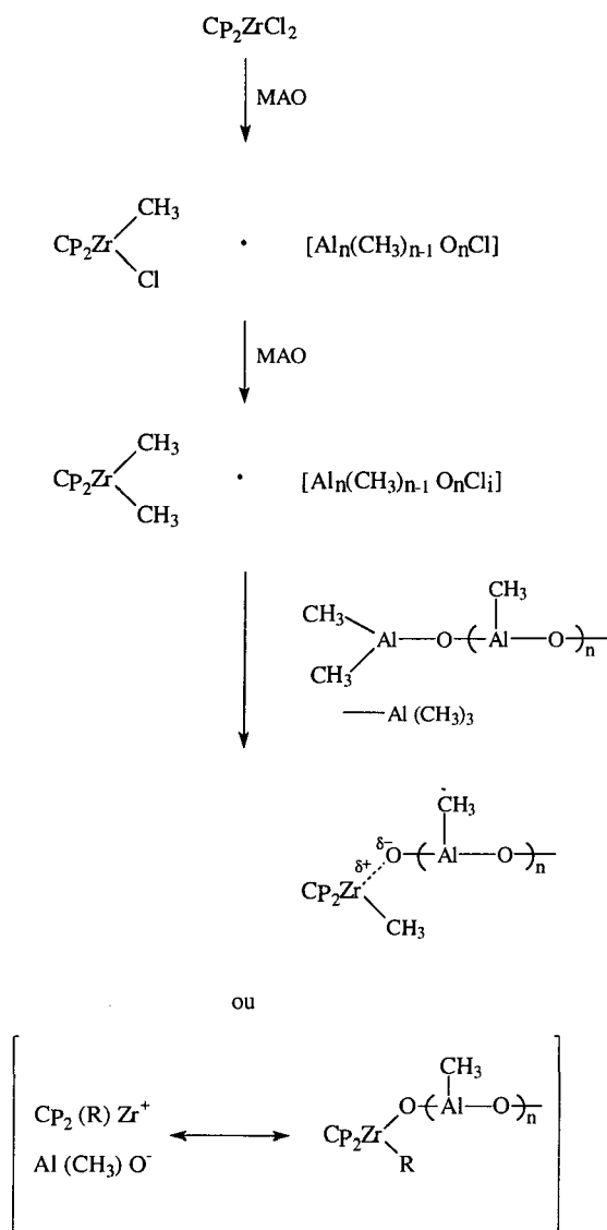
Esquema 1. Formação da espécie ativa [10] nos sistemas metaloceno/MAO
